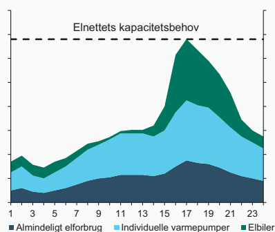
Figur 4.2 Illustrativt eksempel på uflexibelt elforbrug over døgnets timer
