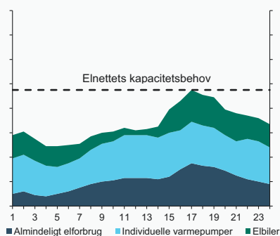
Figur 4.3 Illustrativt eksempel på fleksibelt elforbrug over døgnets timer
